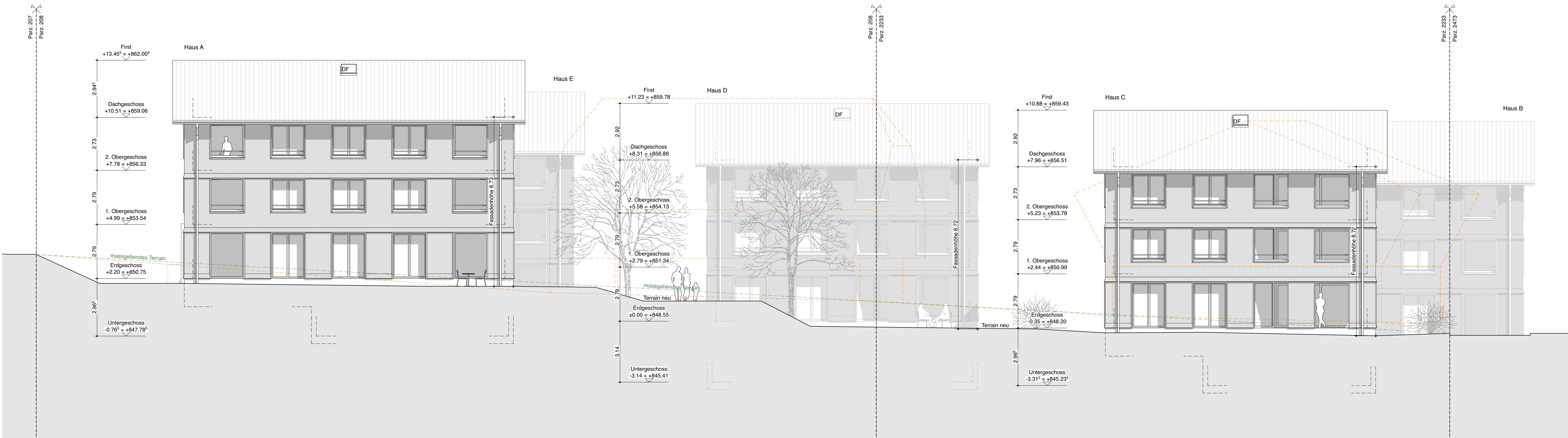
SÜDWESTFASADE
