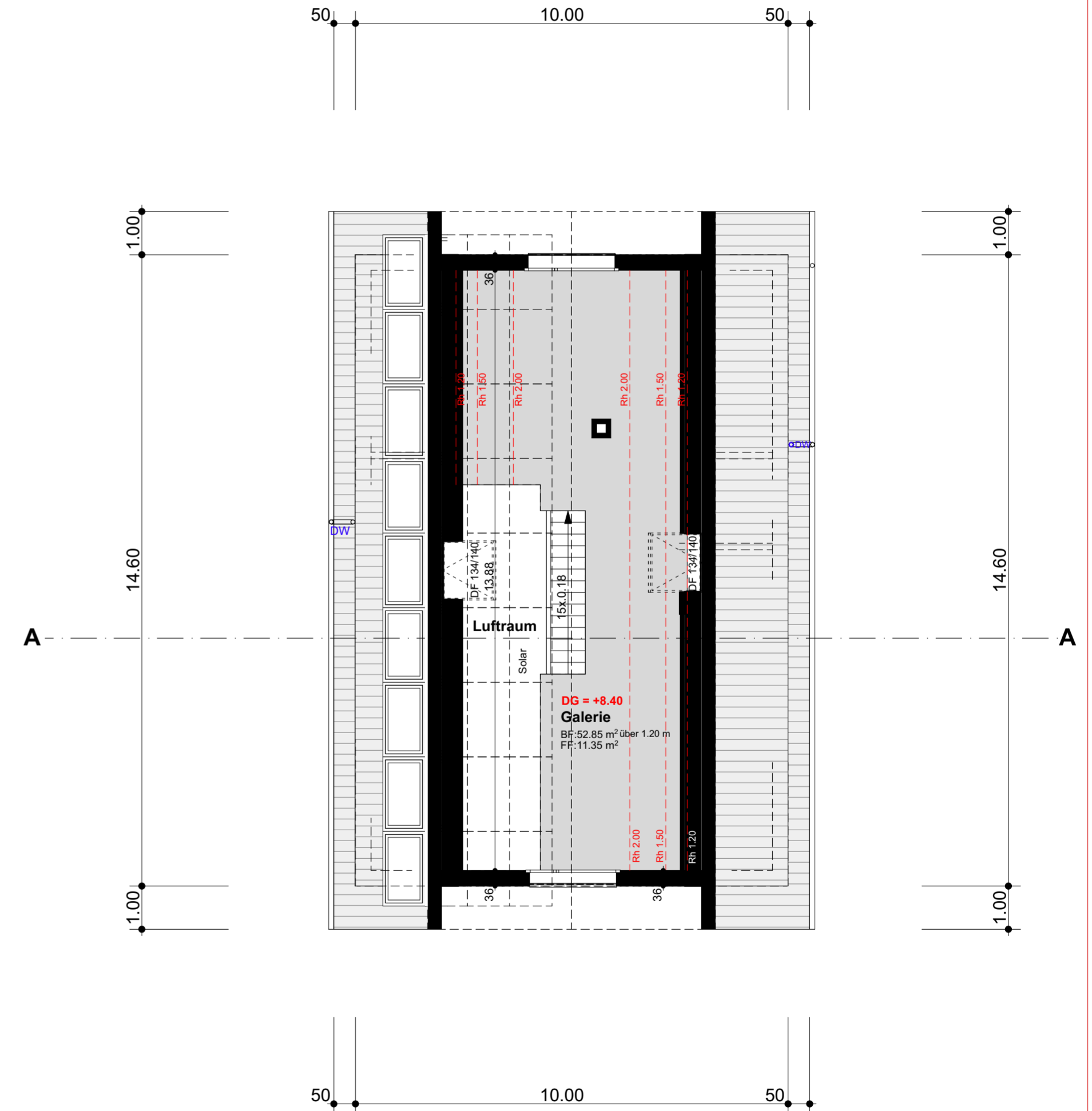
Dachgeschoss
