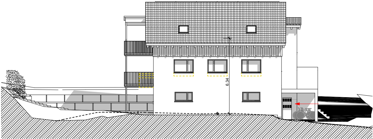
ANSICHT NORDOST
