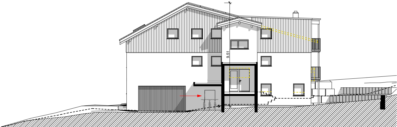
ANSICHT NORDWEST
